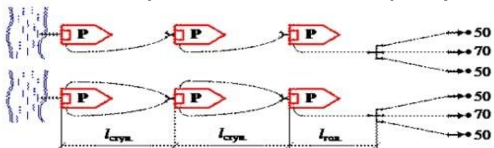
а) из насоса в насос
