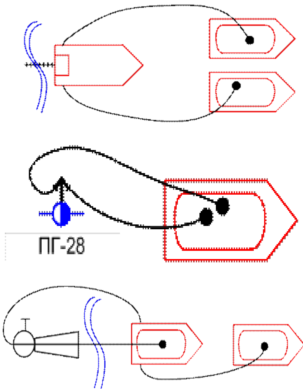
Рисунок 1 - Способы заправки автоцистерн водой при ее подвозе на пожар
