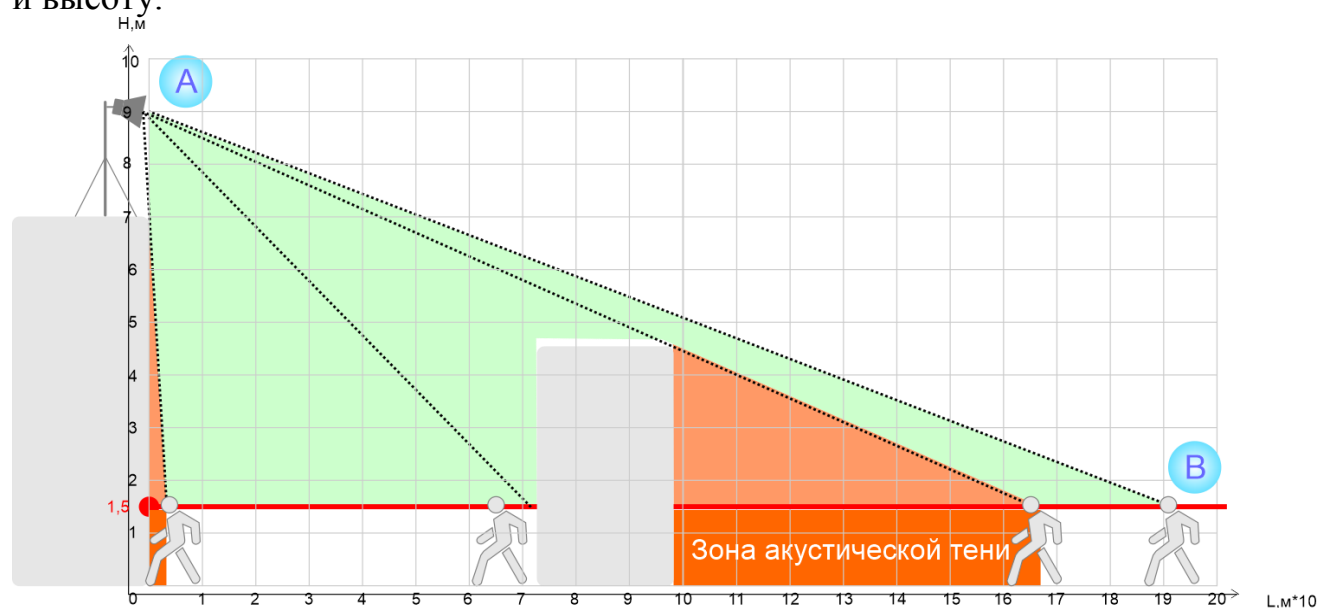
Рис. 9. Влияние на распространение звука, окружающих объект, конструкций, зданий и сооружений.
