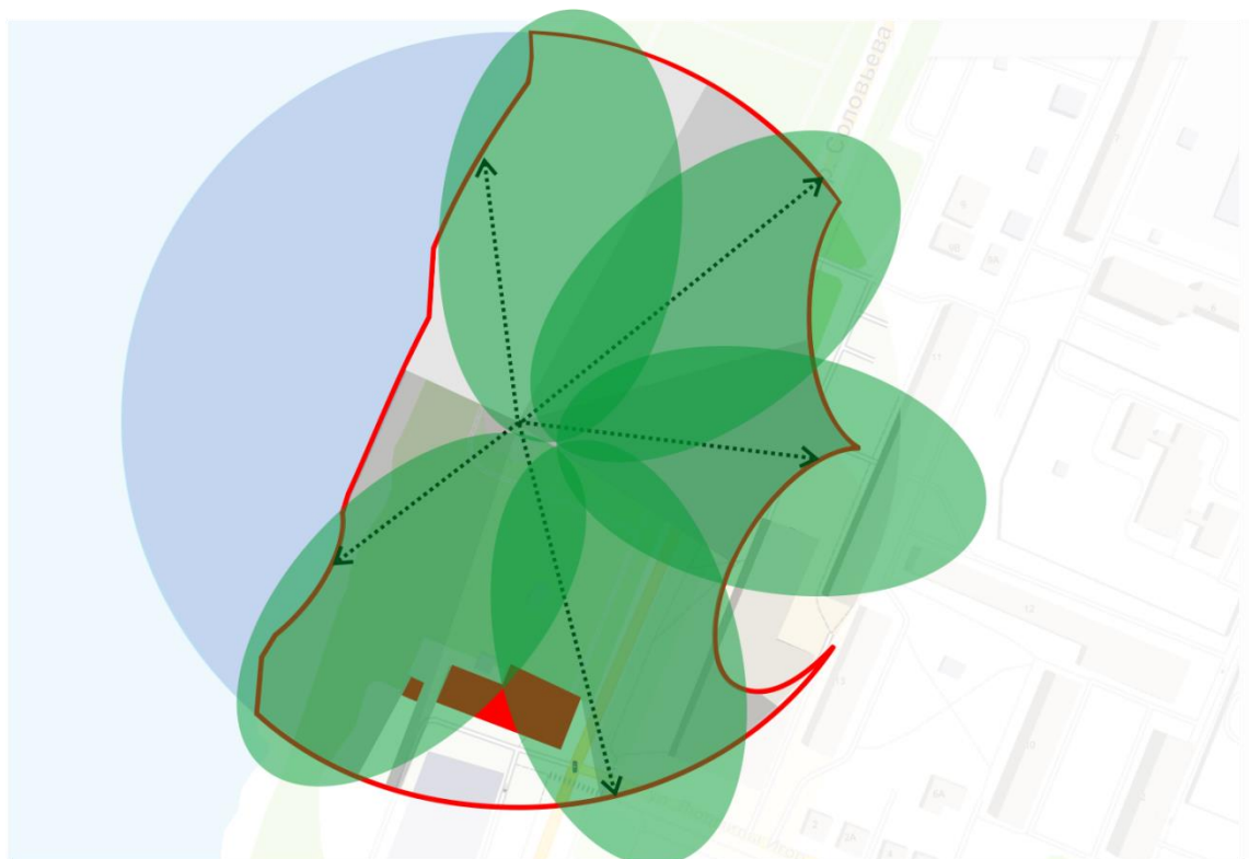
Рис. 7. Зоны покрытия громкоговорителями относительно векторов.
