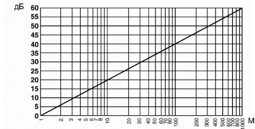
Рис. 12. Зависимость уровня звукового давления громкоговорителя от его удаления.
